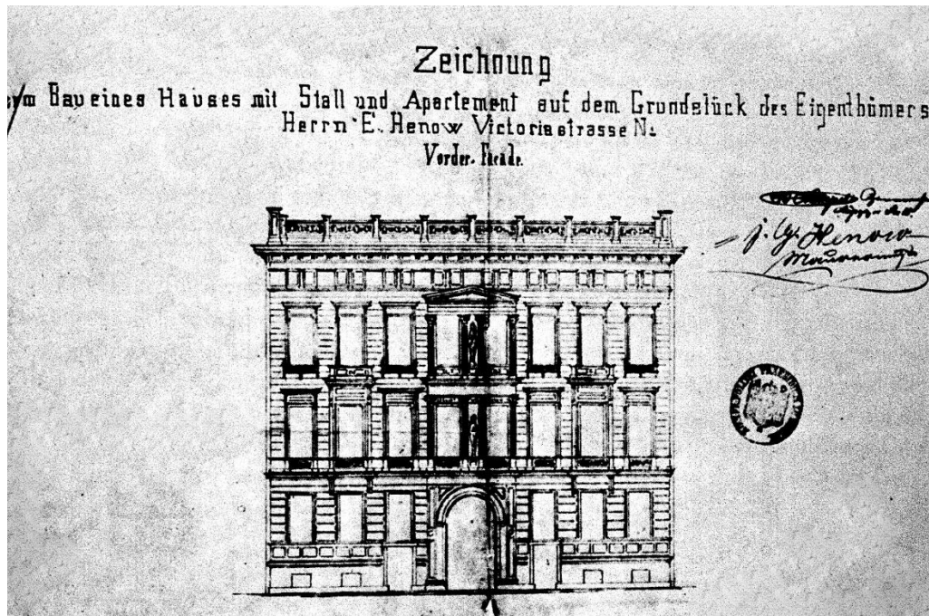
Bauantragszeichnung, Fassade, 1858 aus der Bauakte im Landesarchiv Berlin
