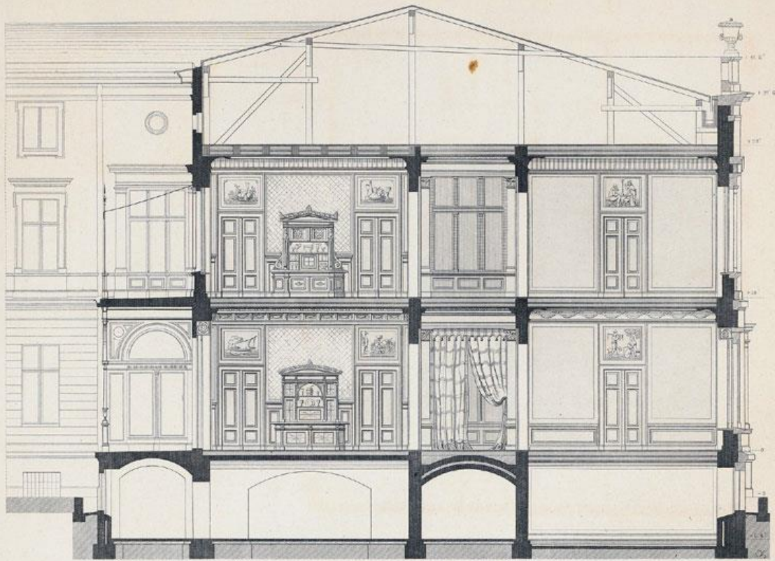
Querschnitt.
